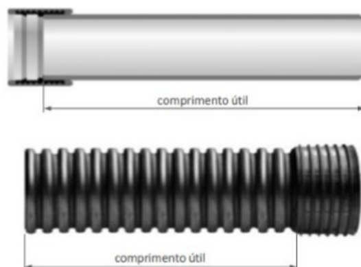
Figura 1 - Rede tubular em PEAD
