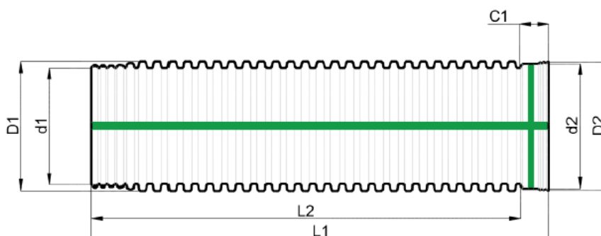
Figura 2 - Imagem ilustrativa de tubulação PEAD
